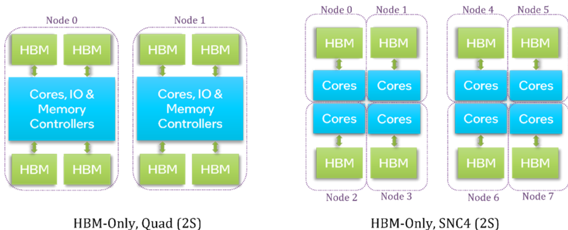
图13. “仅HBM”模式下的NUMA 节点配置
