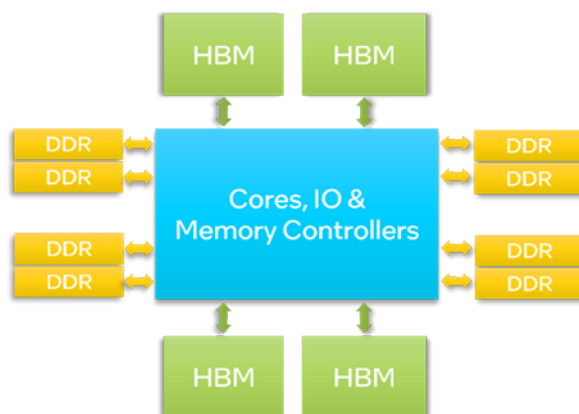
图1. 处理器示意图
